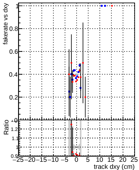
—●— DQM_mkFit_TT_baseline_6iter —●— DQM_mkFit_TT_RetrainV2_WP1_6iter
