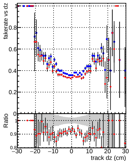
—●— DQM_mkFit_TT_baseline_6iter —●— DQM_mkFit_TT_RetrainV2_WP1_6iter
