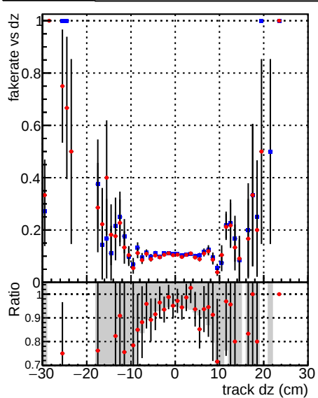
—●— DQM_mkFit_TT_baseline_6iter —●— DQM_mkFit_TT_RetrainV2_WP1_6iter
