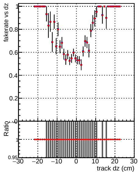
—●— DQM CKF TT_base_noSel —●— DQM CKF TT_baseT125_noSel
