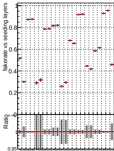
Fake rate vs. —•— DQM CKF TT_base_noSel —•— DQM CKF TT_baseT125_noSel
