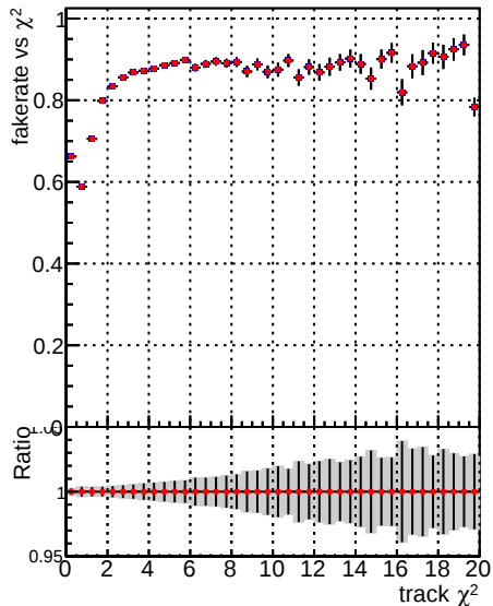
Fake rate vs. —•— DQM CKF TT_base_noSel —•— DQM CKF TT_baseT125_noSel
