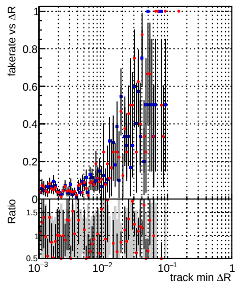
—•— DQM_mkFit_TTbase —•— DQM_mkFit_TT_retrainOldFiles125
