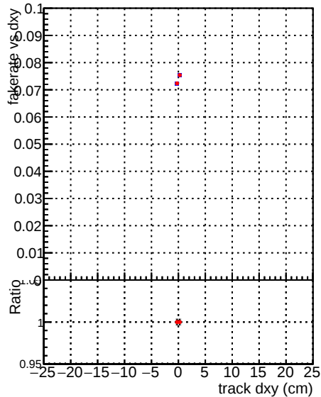
— DQM_mkFit_TTbase — DQM_mkFit_TT_retrainOldFiles125
