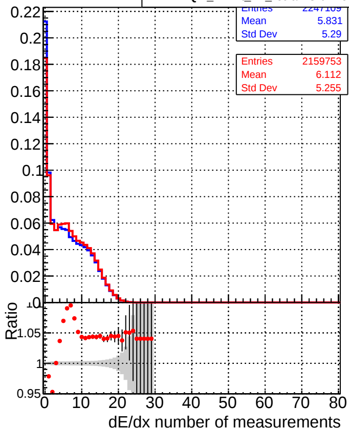
—■— DQM_mkFit_TTbase —●— DQM_mkFit_TT_retrainOldFiles125
