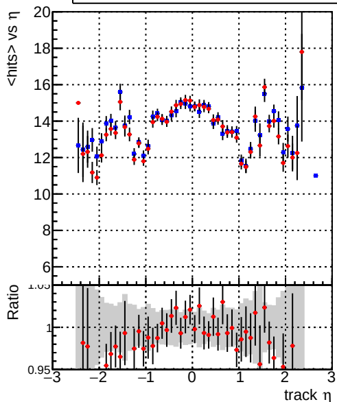
mean hit — DQM_mkFit_TTbase — DQM_mkFit_TT_retrainOldFiles125
