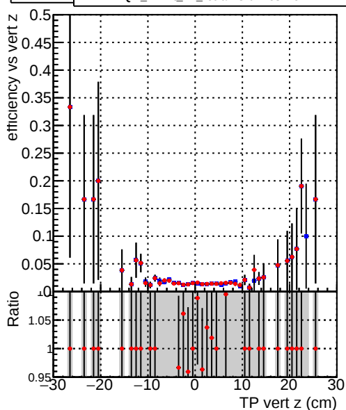
Efficiency —●— DQM_mkFit_TT_retrainOldFiles125
