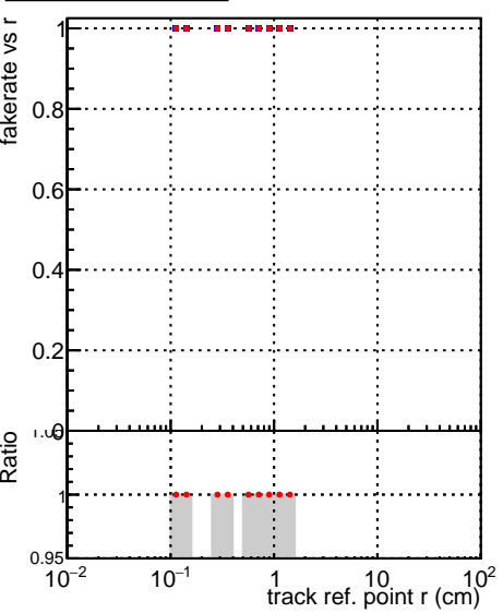
DQM_mkFit_TTbase DQM_mkFit_TT_retrainOldFiles125
