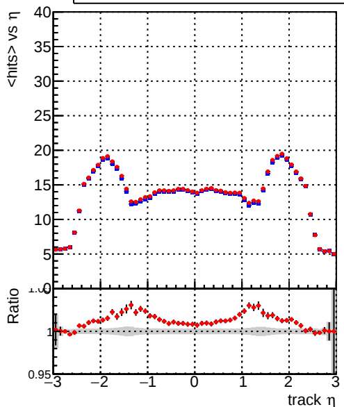
— DQM_mkFit_TTbase — DQM_mkFit_TT_retrainOldFiles125 mean hits
