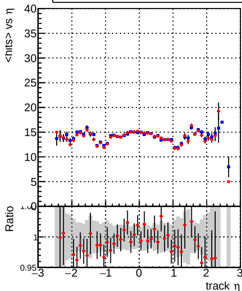
— DQM_mkFit_TTbase — DQM_mkFit_TT_retrainOldFiles125 mean hits
