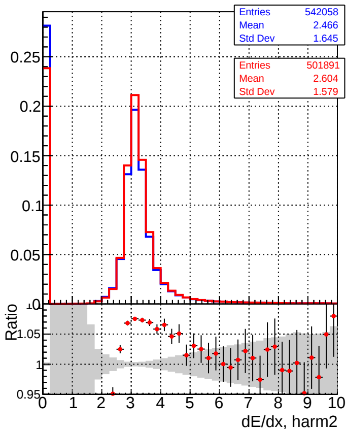
■ DQM_mkFit_TTbase ● DQM_mkFit_TT_retrainOldFiles125
