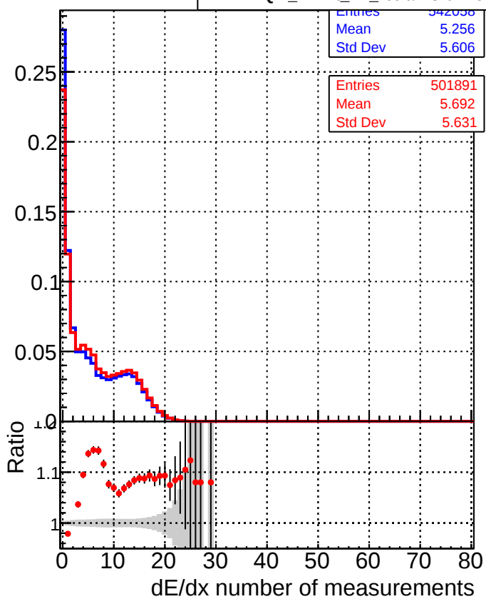
■ DQM_mkFit_TTbase ● DQM_mkFit_TT_retrainOldFiles125
