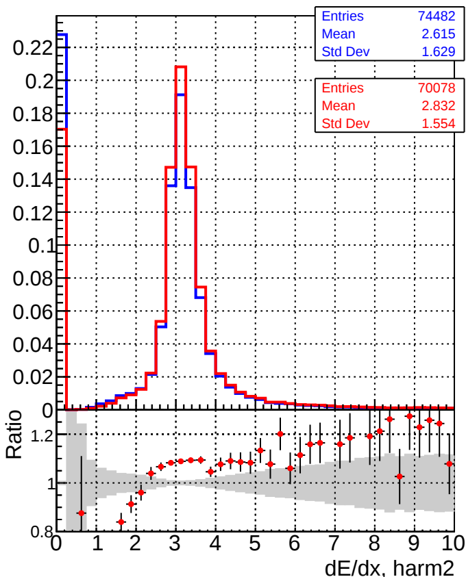
DQM_mkFit_TTbase DQM_mkFit_TT_retrainOldFiles125
