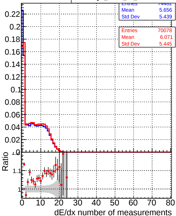
DQM_mkFit_TTbase DQM_mkFit_TT_retrainOldFiles125
