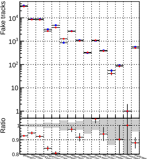
Number —●— DQM_mkFit_TT_retrainOldFiles125
