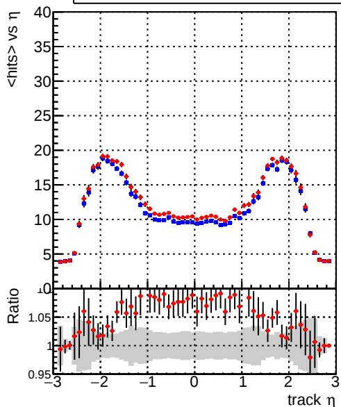
— DQM_mkFit_TTbase — DQM_mkFit_TT_retrainOldFiles125 mean hits
