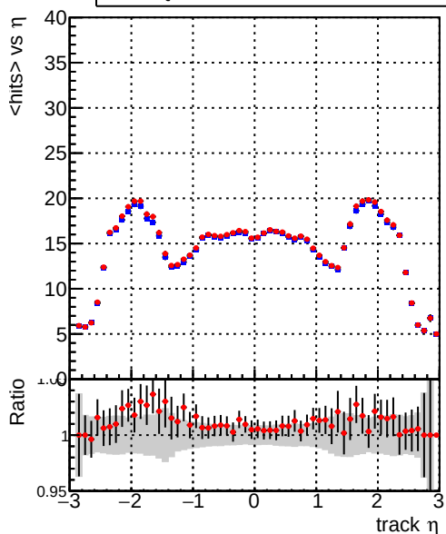
— DQM_mkFit_TTbase — DQM_mkFit_TT_retrainOldFiles125
