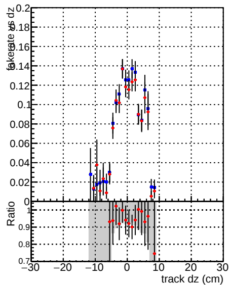
—●— DQM_mkFit_TTbase —●— DQM_mkFit_TT_retrainOldFiles125
