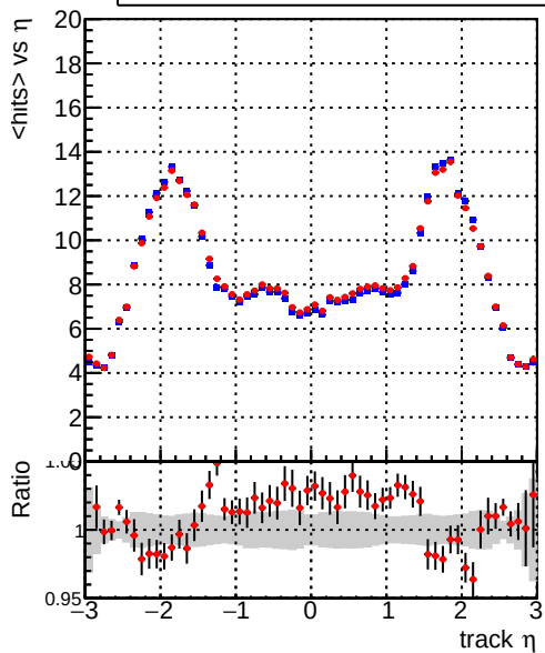
mean hit — DQM_mkFit_TTbase — DQM_mkFit_TT_retrainOldFiles125
