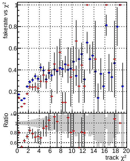
Fake rate vs. —•— DQM mkFit TTbase —•— DQM mkFit TT_retrainOldFiles125
