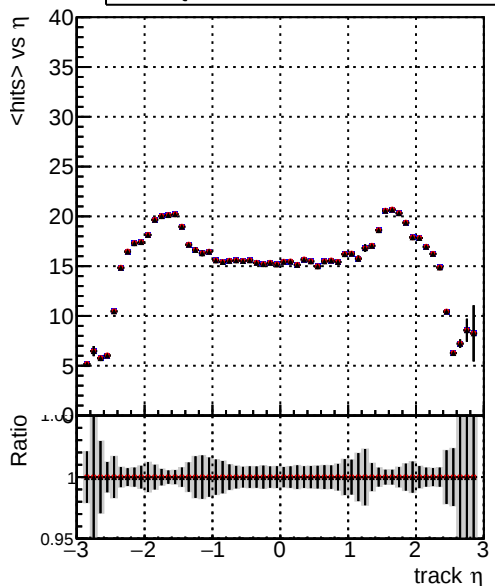
mean hits — DQM_CKF_TT_base_noSel — DQM_CKF_TT_retrainOldFiles113_noSel — DQM_CKF_TT_retrainOldFiles125_noSel
