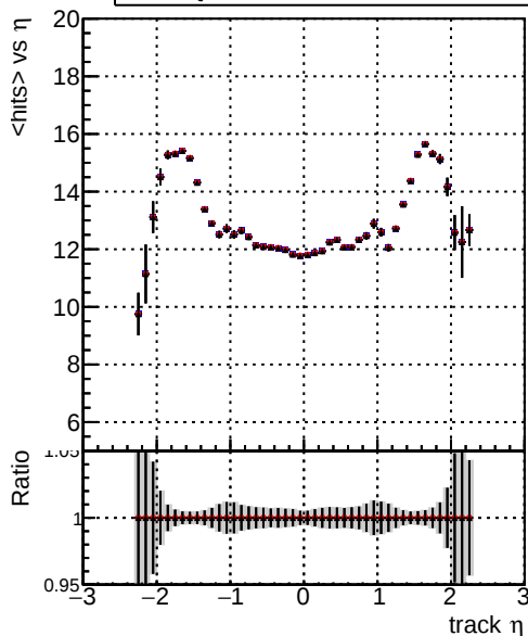
mean hit — DQM_CKF_TT_base_noSel — DQM_CKF_TT_retrainOldFiles113_noSel — DQM_CKF_TT_retrainOldFiles125_noSel
