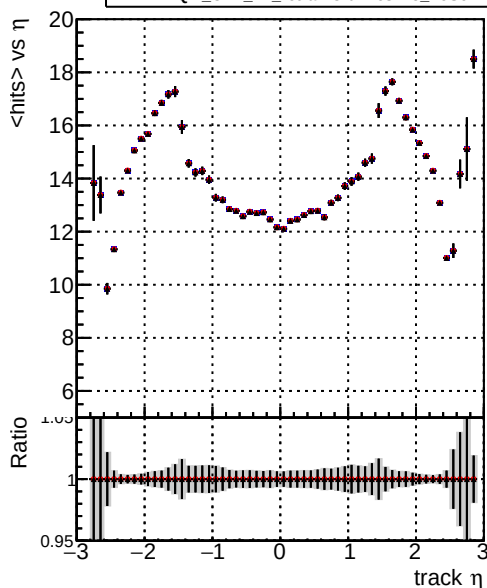
mean hits vs \eta DQM_CKF_TT_base_noSel DQM_CKF_TT_retrainOldFiles113_noSel DQM_CKF_TT_retrainOldFiles125_noSel
