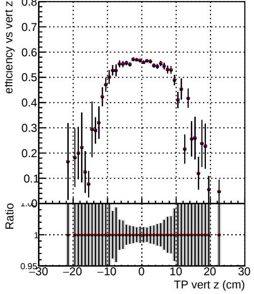
Efficiency vs. TP vert z (cm) —•— DQM_CKF_TT_base_noSel —•— DQM_CKF_TT_retrainOldFiles113_noSel —•— DQM_CKF_TT_retrainOldFiles125_noSel
