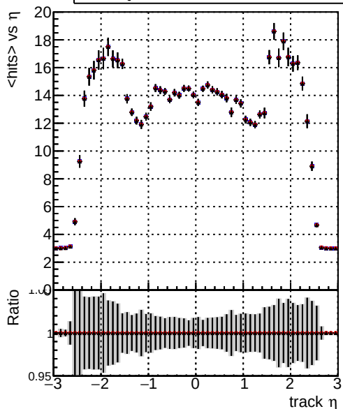
mean hit — DQM_CKF_TT_base_noSel — DQM_CKF_TT_retrainOldFiles113_noSel — DQM_CKF_TT_retrainOldFiles125_noSel
