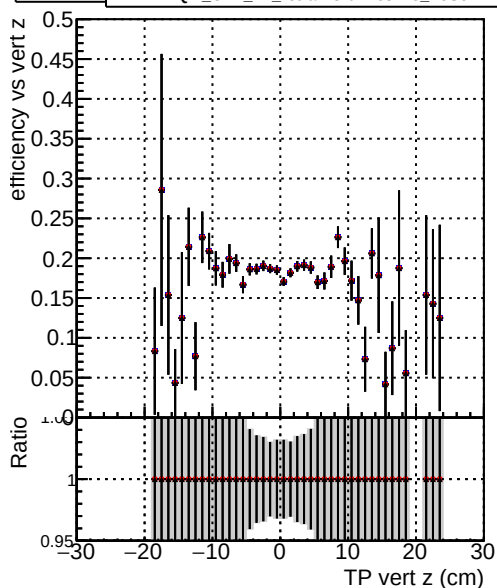
Efficiency vs vert z —•— DQM_CKF_TT_base_noSel —•— DQM_CKF_TT_retrainOldFiles113_noSel —•— DQM_CKF_TT_retrainOldFiles125_noSel
