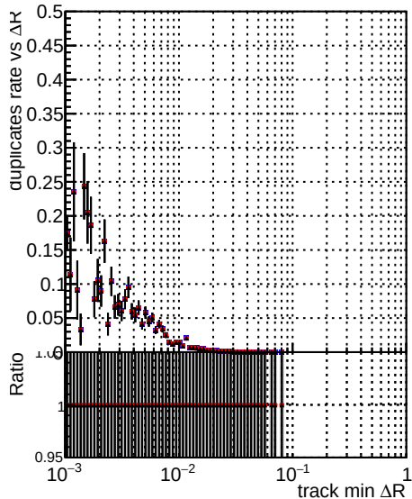
— DOM_CKF_TT_base_noSel — DOM_CKF_TT_retrainOldFiles113_noSel — DOM_CKF_TT_retrainOldFiles125_noSel
