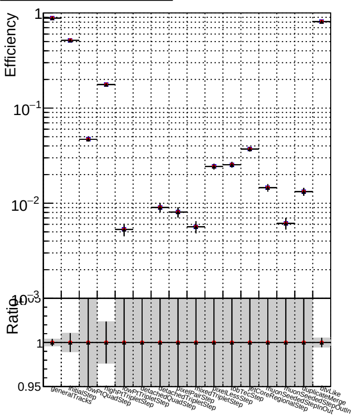
DQM_CKF_TT_base_noSel DQM_CKF_TT_retrainOldFiles113_noSel DQM_CKF_TT_retrainOldFiles125_noSel
