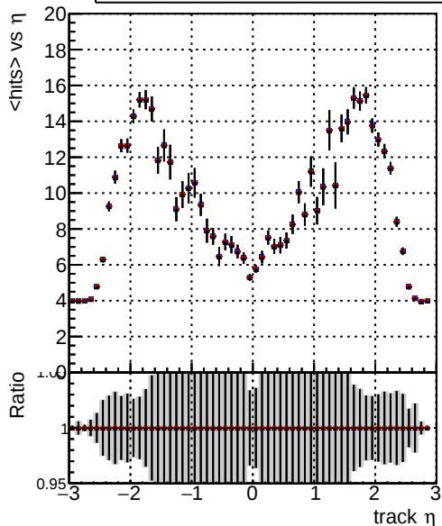
mean hits — DQM_CKF_TT_base_noSel — DQM_CKF_TT_retrainOldFiles113_noSel — DQM_CKF_TT_retrainOldFiles125_noSel
