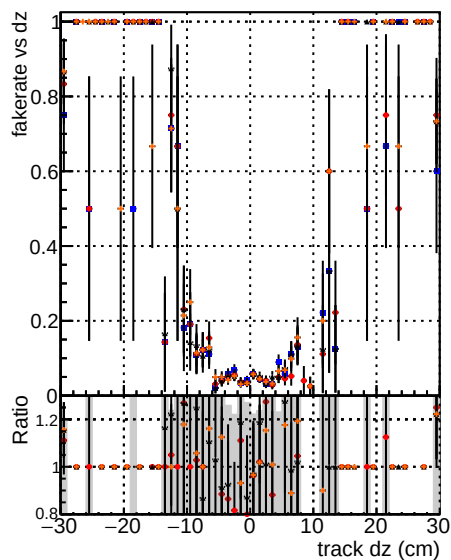
Fake rate vs dz DGM mkt Fit TTbase DGM mkt Fit TrainOldFiles125 DGM mkt Fit TrainNewFiles125 AndSQCD
