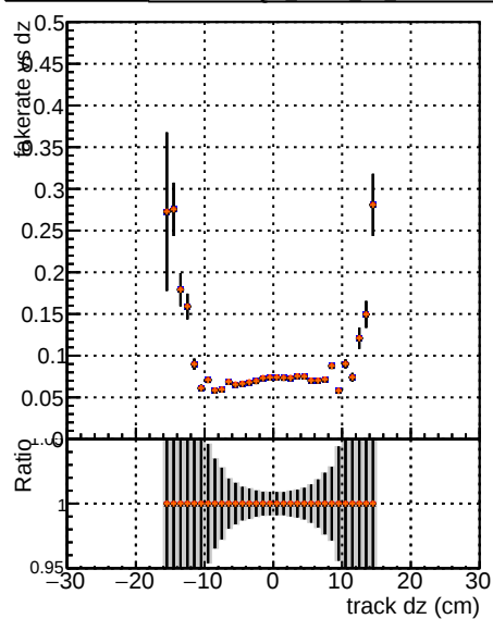
Legend: DOM mkrFit TTbase DOM mkrFit TTbaseAndSQCD DOM mkrFit TTbaseAndSQCD
