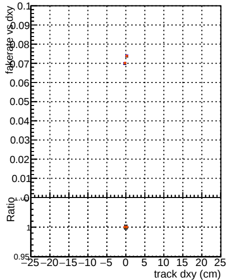
Legend: DOM mkrFit TTbase DOM mkrFit TTbaseAndSQCD DOM mkrFit TTbaseAndSQCD
