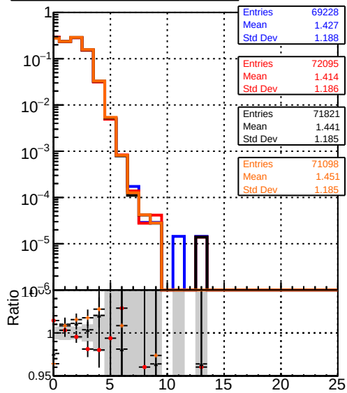
DQM_mkFit_TTbase DQM_mkFit_TT_retrainOldFiles125 DQM_mkFit_TT_retrainNewFiles125 DQM_mkFit_TT_retrainNewFiles125AndSQCD mean hit
