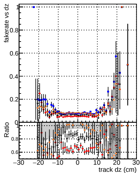
Fake rate vs dz DQM mkFit TTbase DQM mkFit TTbase TrainNewFiles125 DQM mkFit TTbase TrainNewFiles125 AndSQCD
