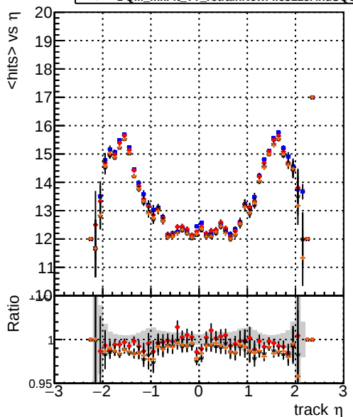
mean hit DQM_mkFit_TTbase DQM_mkFit_TT_retrainOldFiles125 DQM_mkFit_TT_retrainNewFiles125 DQM_mkFit_TT_retrainNewFiles125AndSQCD
