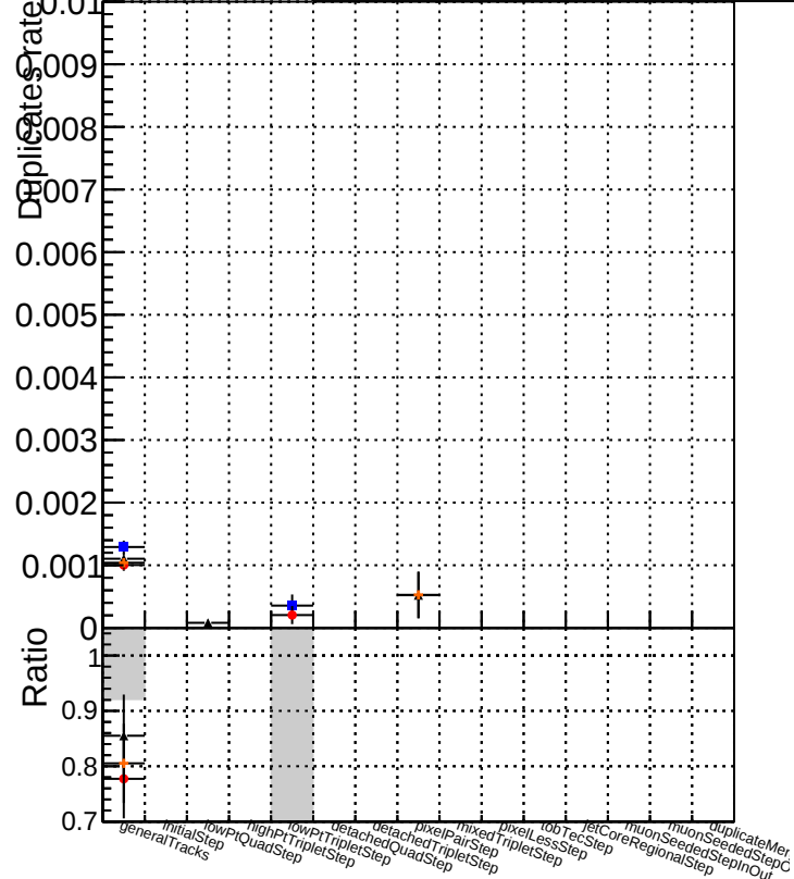
Duplicates rate vs collection Legend: DQM_mkFit_TTbase DQM_mkFit_TT_retrainOldFiles125 DQM_mkFit_TT_retrainNewFiles125 DQM_mkFit_TT_retrainNewFiles125AndSQCD
