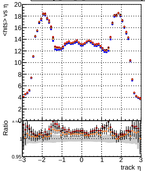
DQM_mkFit_TTbase DQM_mkFit_TT_retrainOldFiles125 DQM_mkFit_TT_retrainNewFiles125 DQM_mkFit_TT_retrainNewFiles125AndSQCD mean hit
