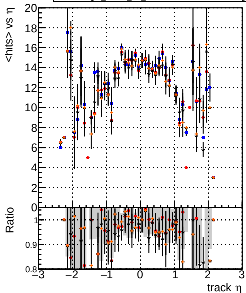
— DQM_mkFit_TTbase — DQM_mkFit_TT_retrainOldFiles125 — DQM_mkFit_TT_retrainNewFiles125 — DQM_mkFit_TT_retrainNewFiles125AndSQCD mean hit
