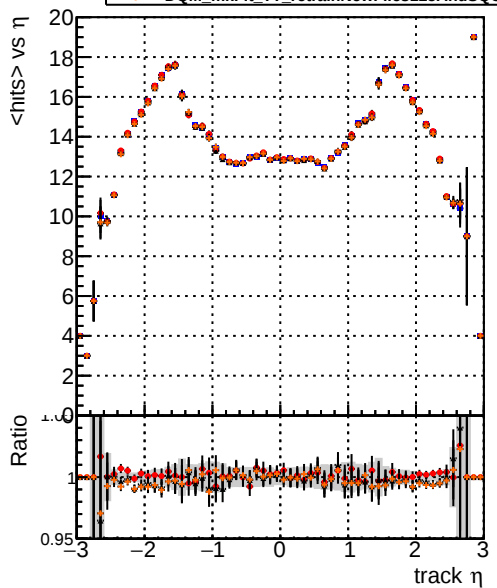
mean hits vs \eta DQM_mkFit_TTbase DQM_mkFit_TT_retrainOldFiles125 DQM_mkFit_TT_retrainNewFiles125 DQM_mkFit_TT_retrainNewFiles125AndSQCD
