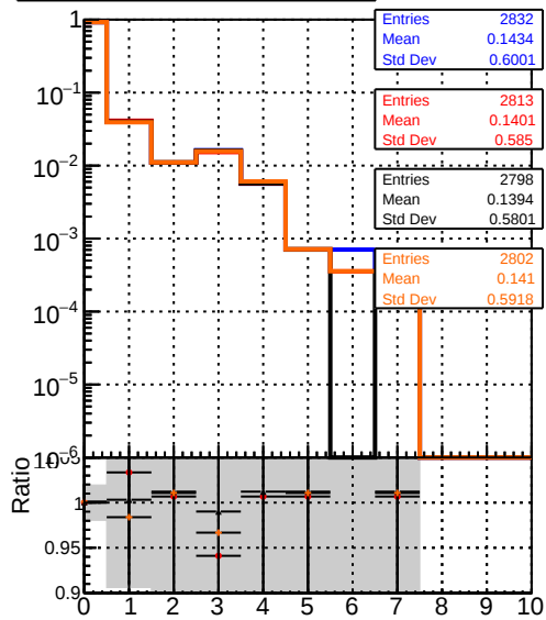
mean hits DQM_mkFit_TTbase DQM_mkFit_TT_retrainOldFiles125 DQM_mkFit_TT_retrainNewFiles125 DQM_mkFit_TT_retrainNewFiles125AndSQCD
