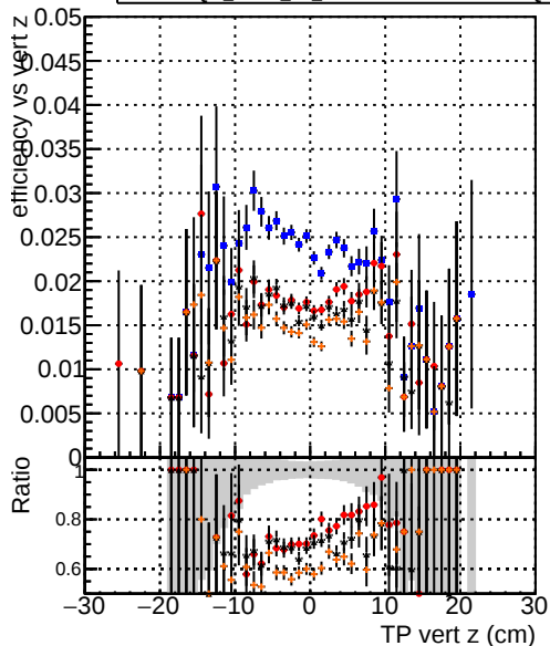
Efficiency —●— DQM_mkFit_TT_retrainOldFiles125 —★— DQM_mkFit_TT_retrainNewFiles125 —+— DQM_mkFit_TT_retrainNewFiles125AndSQCD
