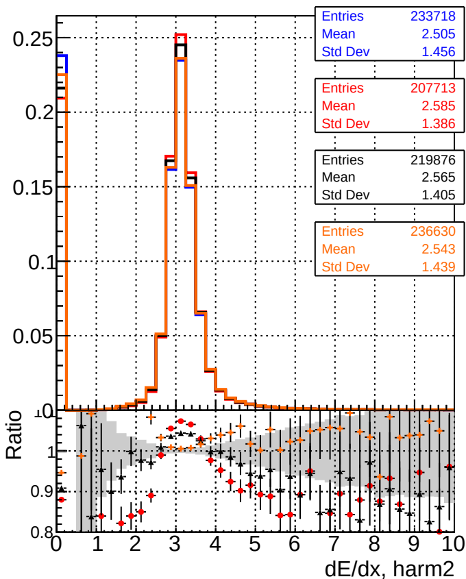
— DQM_mkFit TTbase — DQM_mkFit TT_retrainOldFiles125 — DQM_mkFit TT_retrainNewFiles125 — DQM_mkFit TT_retrainNewFiles125AndSQCD
