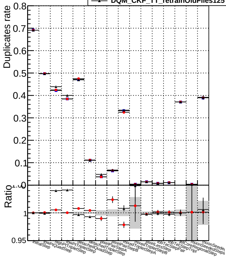
Duplicates rate vs c ● DQM_CKF_TT_retrainOldFiles113 ▲ DQM_CKF_TT_retrainOldFiles125
