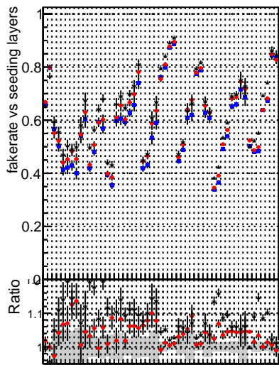
Fake rate vs. —●— DGM CKF TTbase —●— DGM CKF TTbase retrainOldFiles113
