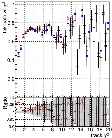
Fake rate vs. —●— DGM CKF TTbase —●— DGM CKF TTbase retrainOldFiles113
