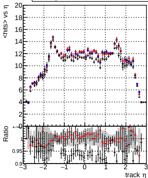
mean hits vs \eta — DQM_CKF_TTbase — DQM_CKF_TT_retrainOldFiles113 — DQM_CKF_TT_retrainOldFiles125
