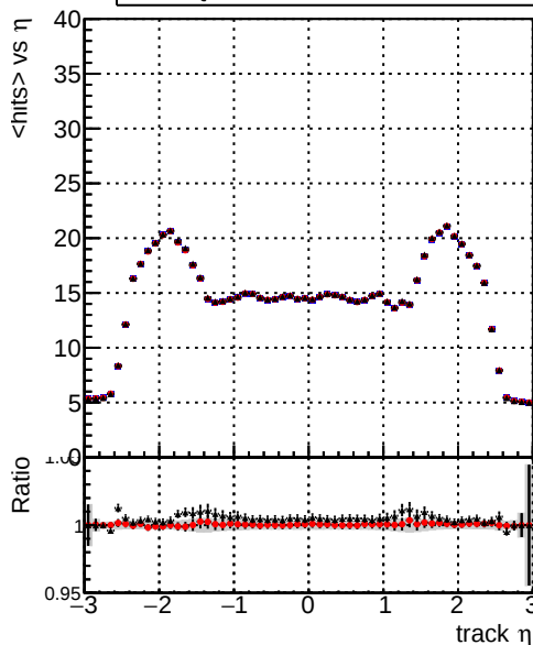
— DQM_CKF_TTbase — DQM_CKF_TT_retrainOldFiles113 — DQM_CKF_TT_retrainOldFiles125 mean hits
