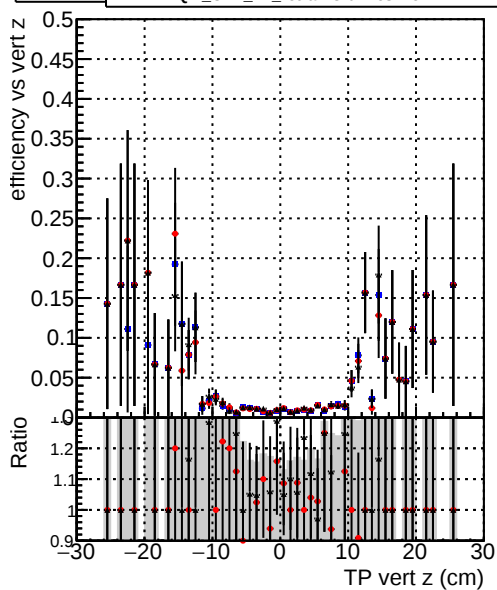
Efficiency vs. TP vert z (cm) — DQM_CKF_TTbase — DQM_CKF_TT_retrainOldFiles113 — DQM_CKF_TT_retrainOldFiles125
