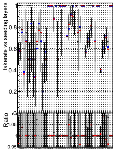
Fake rate vs. DGM CKF TTbase DGM CKF retrainOldFiles123
