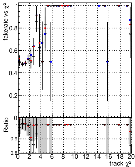
Fake rate vs. DGM CKF TTbase DGM CKF retrainOldFiles123
