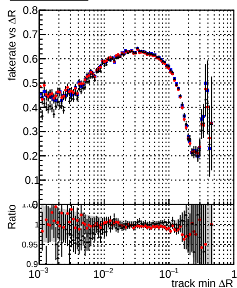
—●— DQM_CKF_TTbase —●— DQM_CKF_TT_retrainOldFiles113 —●— DQM_CKF_TT_retrainOldFiles125
