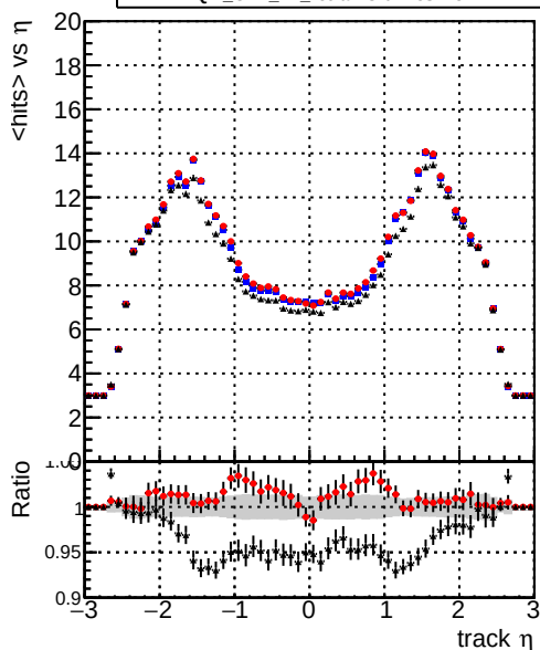
mean hits DQM_CKF_TTbase DQM_CKF_TT_retrainOldFiles113 DQM_CKF_TT_retrainOldFiles125
