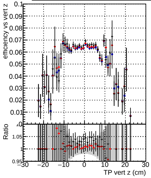
Efficiency vs. TP vert z —●— DQM_CKF_TTbase —●— DQM_CKF_TT_retrainOldFiles113 —●— DQM_CKF_TT_retrainOldFiles125
